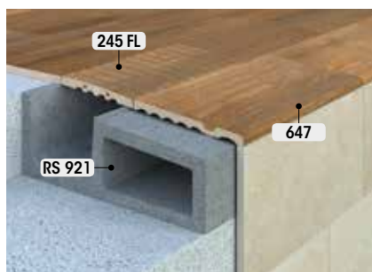
245 FL anti-slip 24,5 x 49,5 x 2,2
