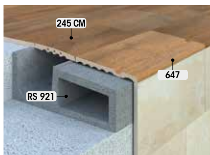
245 CM anti-slip 24,5 x 62,6 x 2,2
