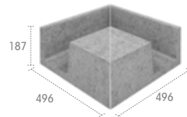
RS 903 Esquina Interior Inside corner Angle intérieur
